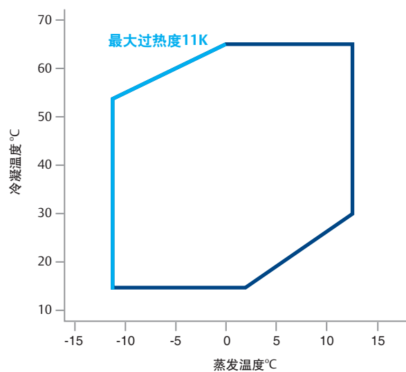
ZB95KQ/ZB114KQ (TW7, TW5 电机)
