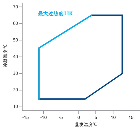
ZB95KQ/ZB114KQ (仅适用于TFD电机)
