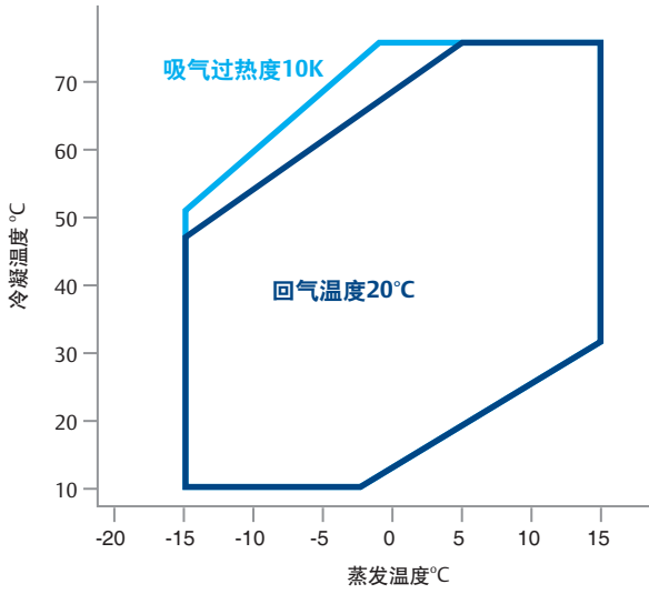
ZB95KQE/ZB114KQE(仅适用于TFD电机)
